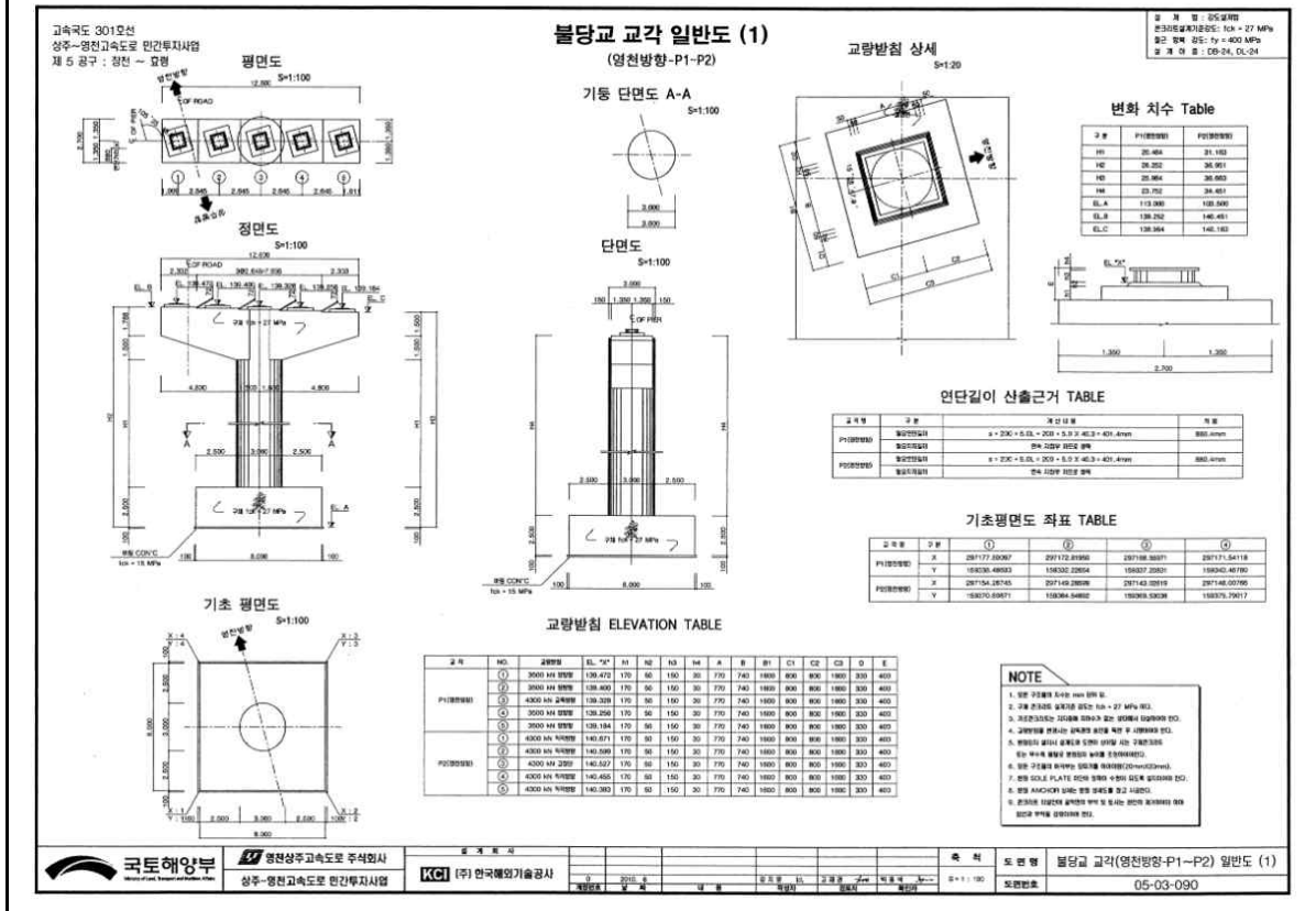
【그림 13.1.7】 교각 일반도
