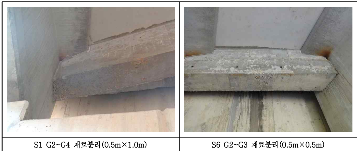
【사진 13.3.7】 가로보 손상현황
